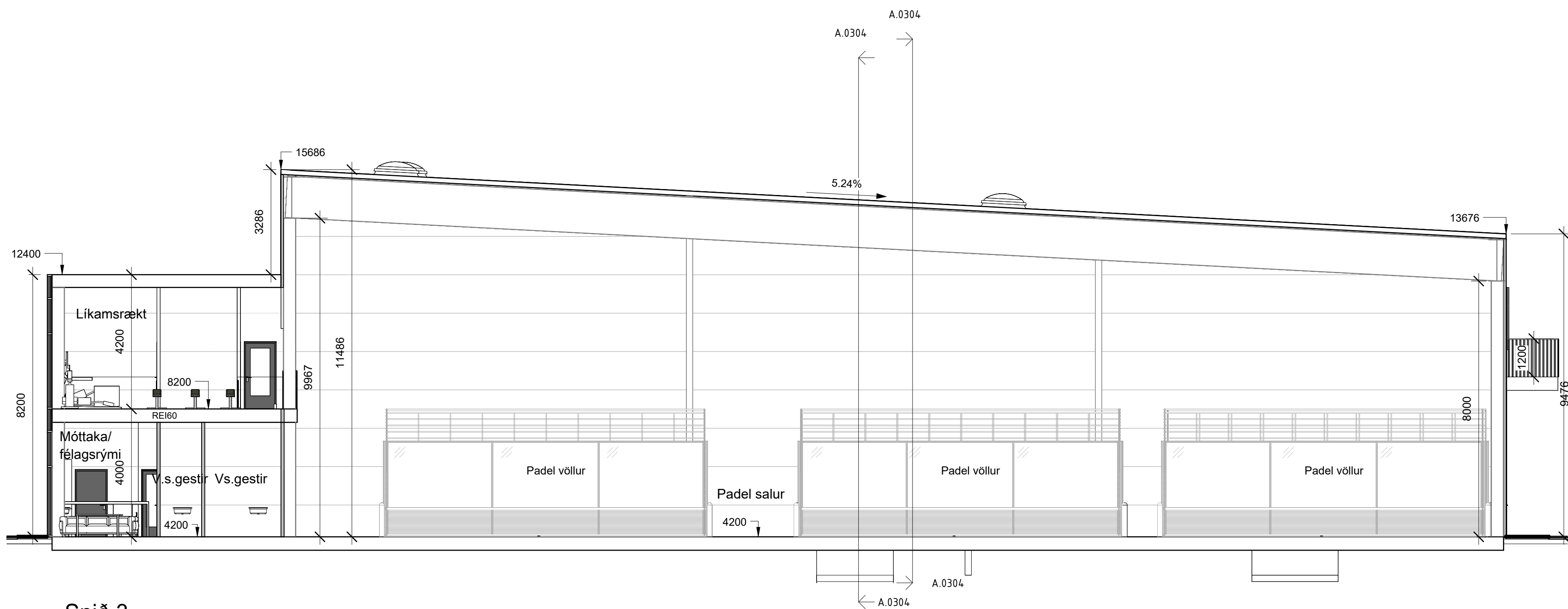
Snið 3 1 : 100
